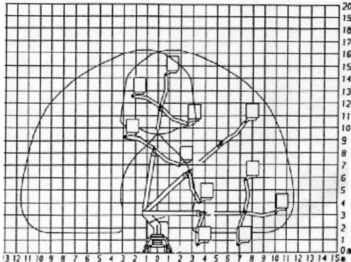
Reichweiten- und Traglastdiagramm
