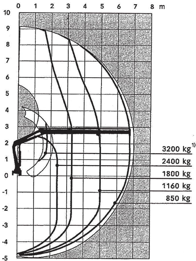
Reichweiten- und Traglastdiagramm
